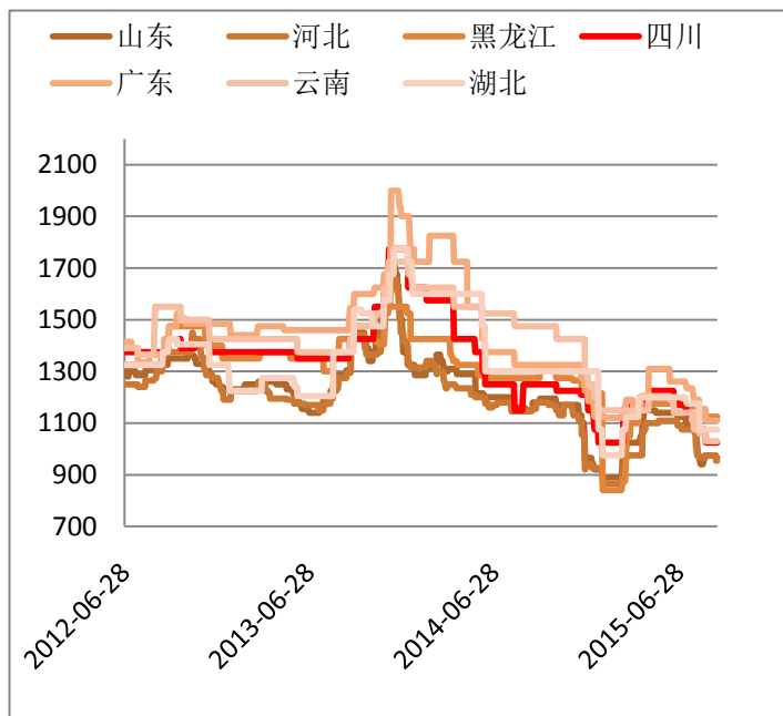
图表 4 甲醛
