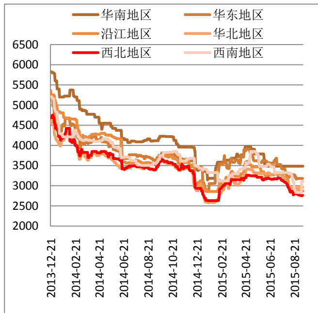
图表 5. 二甲醚
